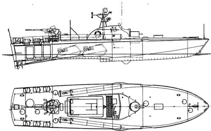
Arrangemangsrättning för Mtb typ T32. Kockums 1951.
